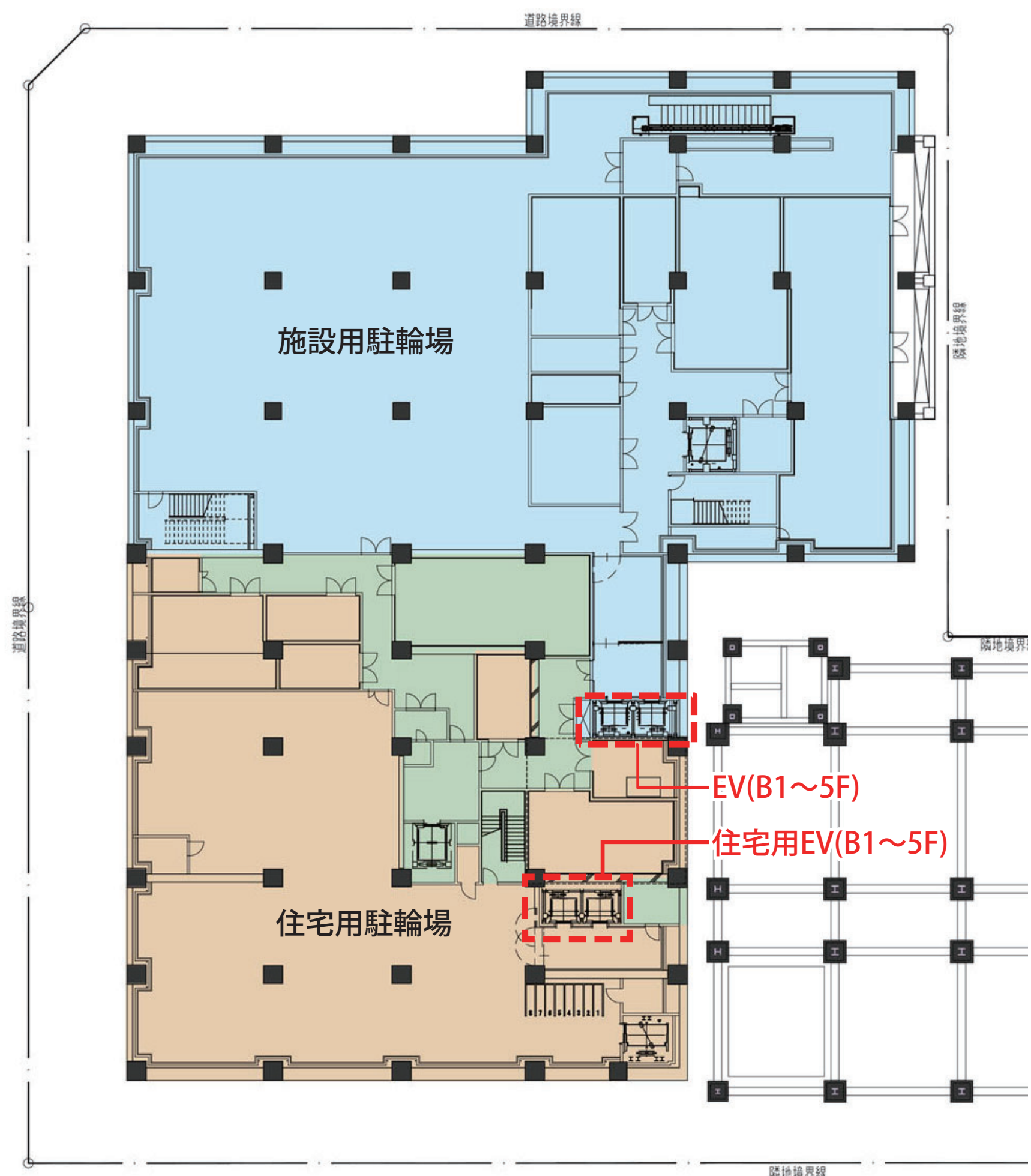
地下1階平面図
